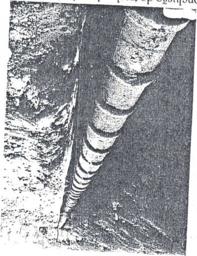
Conclusão de tacho da rede de água pluvial
